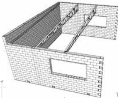
Paneles de dinteles de antepechos para abertura
